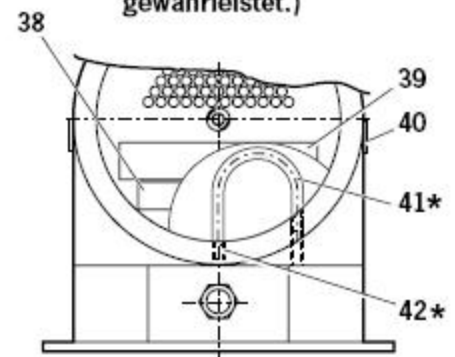
ANSICHT AUF PFEIL "B"
