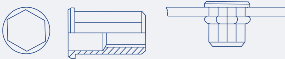
Grip-Sert® Sechskantschaft mit Flachkopf
