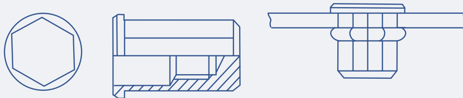
Grip-Sert® Sechskantschaft mit Flachkopf geschlossen
