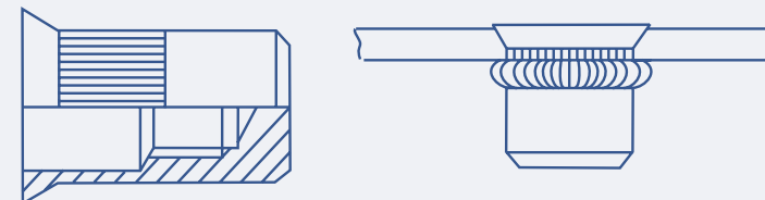
Grip-Sert® Senkkopf Rändelschaft geschlossen
