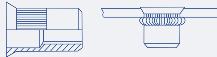
Grip-Sert® Senkkopf Rändelschaft
