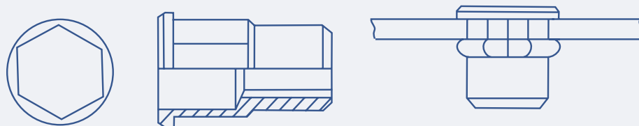
Grip-Sert® Teilsechskantschaft mit Flachkopf
